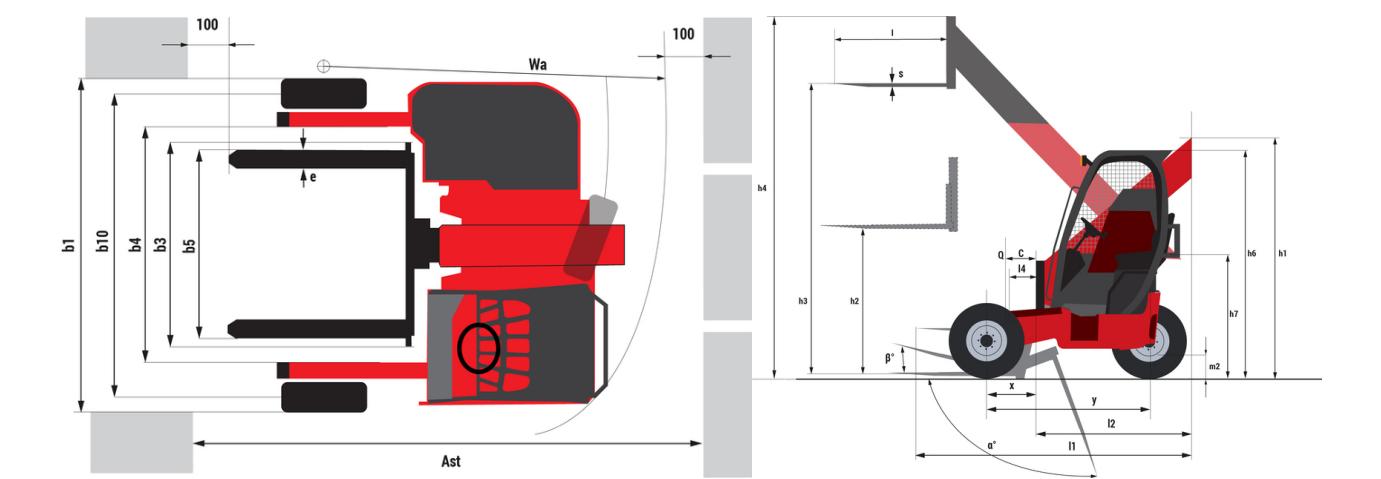
TMT 27P Y ST5 - Maßzeichnung
