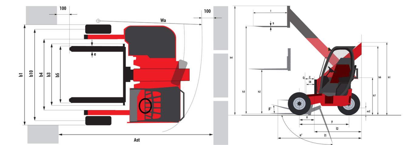
TMT 25 S Y ST5 - Maßzeichnung
