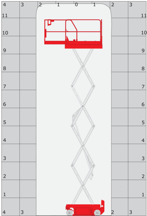
Lastdiagramm
